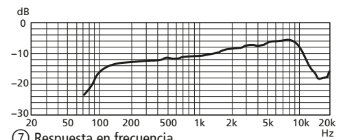
7 Respuesta en frecuencia
