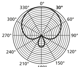
8 Charakterystyka kierunkowości w poziomie
