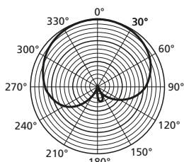
9 Charakterystyka kierunkowości w pionie
